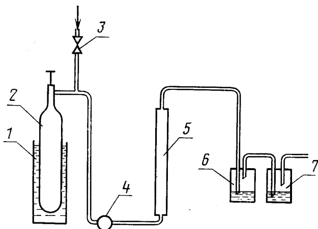
Схема установки для отбора аналитических навесок дихлорсилана
