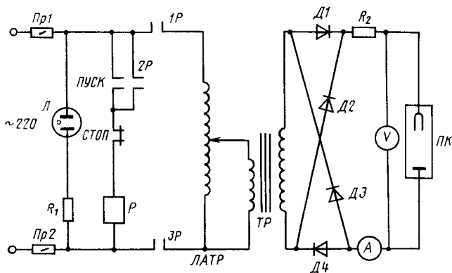
Схема электропитания установки полого катода
