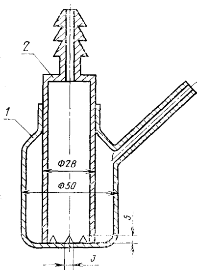
1—полиэтиленовая банка БЦ-100; 2—цилиндр из фторопласта
